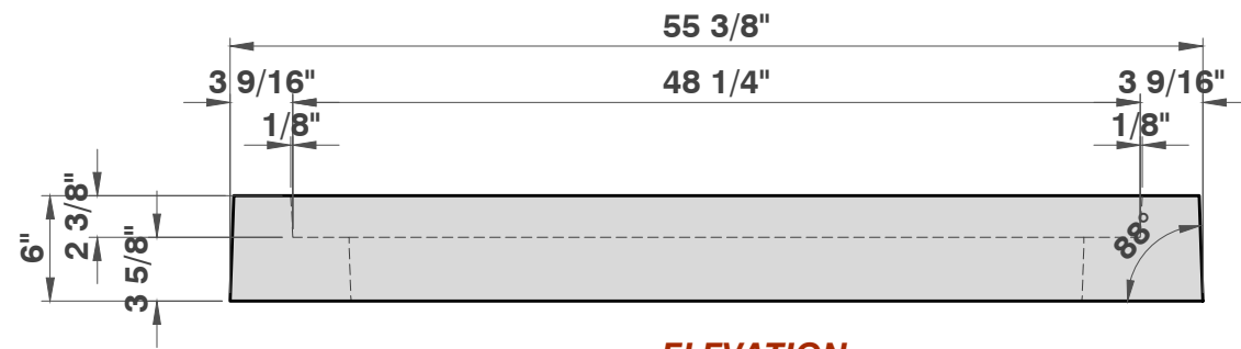
ELEVATION 1"=1'
