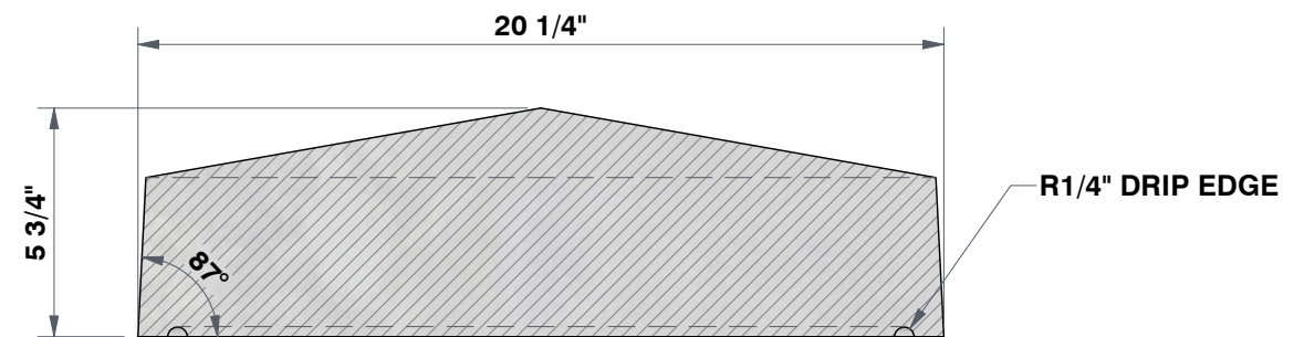
SECTION A-A 2 1/4"=1'
