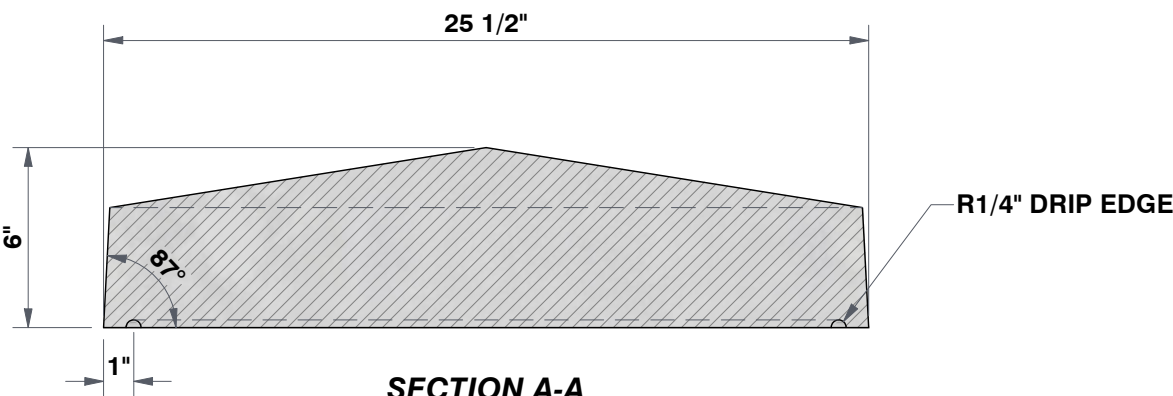
SECTION A-A 1 7/8"=1'
