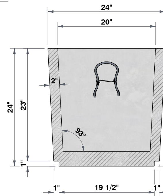
SECTION A-A 1 1/16"=1'
