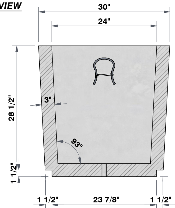
SECTION A-A 7/8"=1'
