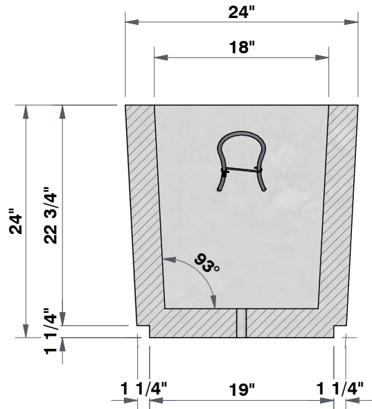
SECTION A-A 7/8"=1'
