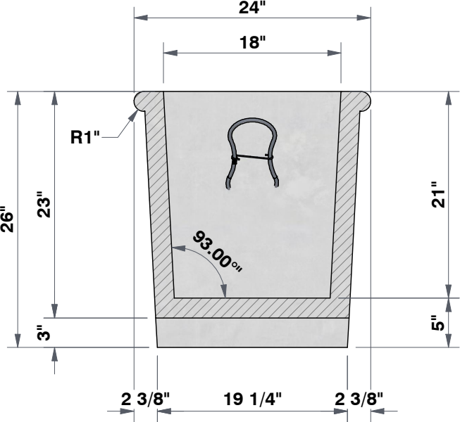
SECTION A-A 7/8"=1'
