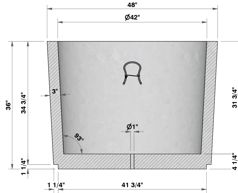
SECTION A-A 7/8"=1'
