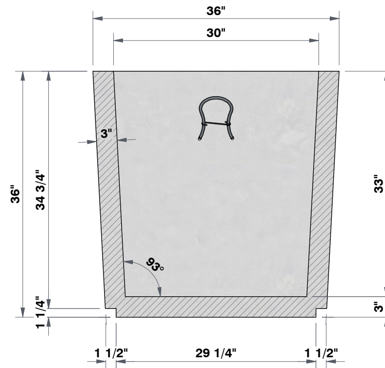
SECTION A-A 7/8"=1'
